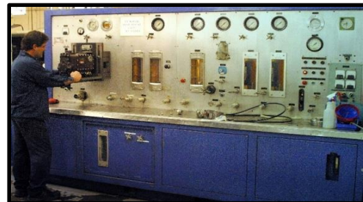
BANCOS DE PRUEBA DE CARGA HIDRÁULICA
