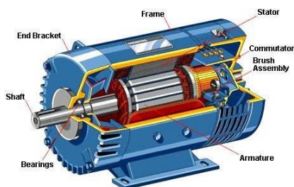
Desintegración del Motor DC
