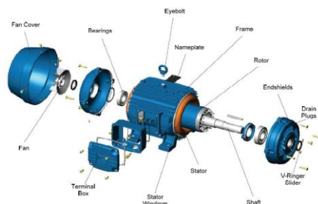
Desintegración del Motor AC
