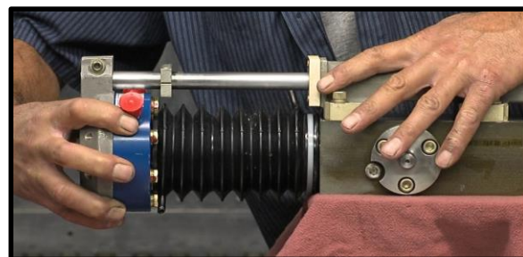
Actuador de Posición Hidráulico
